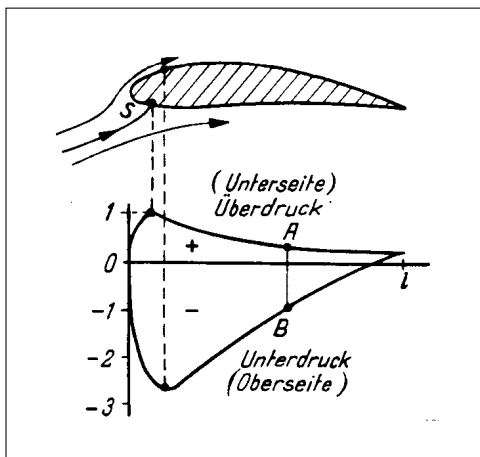
L'aérodynamique d'une aile
